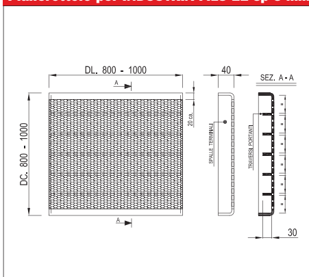
Pianerottolo per INDUSTRIA FILS 21 sp 3 mm
